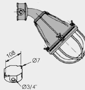
AY40/_P90 - Poste 90°
