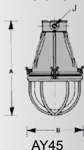
Plafonier
