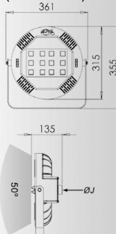
ALEDZCnC3 (100 a 145W)
