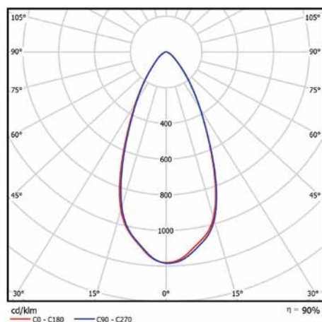
LED 36W - Lente 50° e 100°
